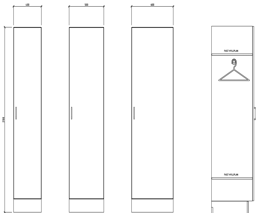
GARDEROB BGS400V/H ART. NR. 318364-0 (V) ART. NR. 318364-1 (H) ART. NR. 318364-0-12 (V) ART. NR. 318364-1-12 (H)
