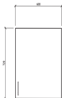
VÄGGSKÅP BVST600V/H ART. NR. 318206-0 (V) ART. NR. 318206-1 (H) ART. NR. 318206-0-12 (V) ART. NR. 318206-1-12 (H)
