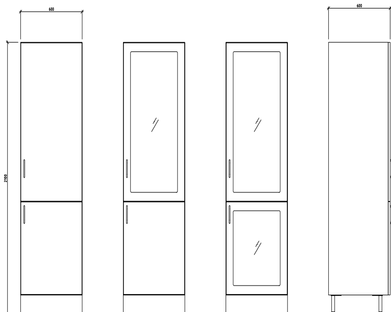
HÖGSKÅP BHSTD600V/H ART. NR. 318336-0 (V) ART. NR. 318336-1 (H) ART. NR. 318336-0-12 (V) ART. NR. 318336-1-12 (H)
