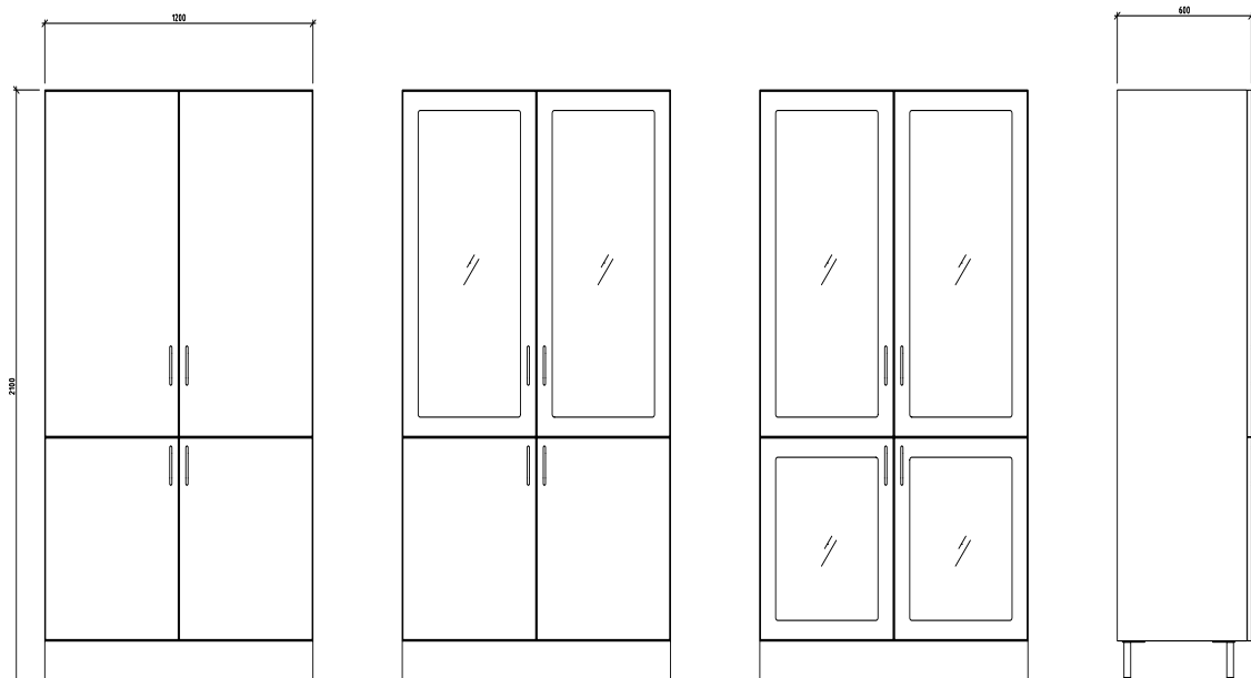
HÖGSKÅP BHSTD1200 ART. NR. 3183312 ART. NR. 3183312-12
