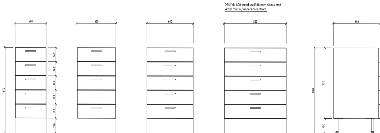
BÄNKSÅP BLH405 ART. NR. 318114-5 ART. NR. 318114-5-12
