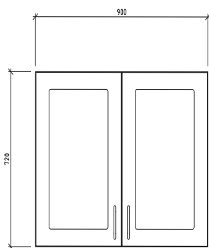
VÄGGSKÅP BVSG900 ART. NR. 318219 ART. NR. 318219-12
