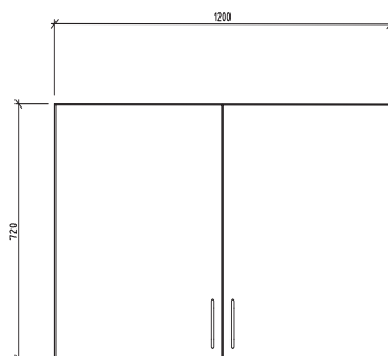
VÄGGSKÅP BVST1200 ART. NR. 3182012 ART. NR. 3182012-12
