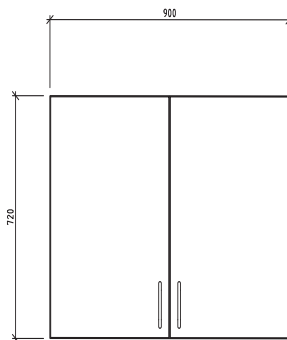
VÄGGSKÅP BVST900 ART. NR. 318209 ART. NR. 318209-12
