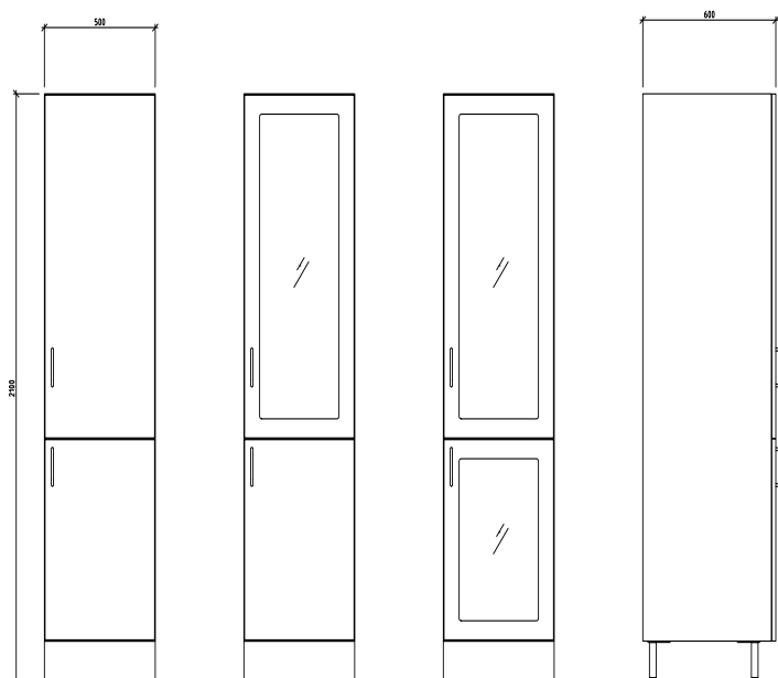
HÖGSKÅP BHSTD500V/H ART. NR. 318335-0 (V) ART. NR. 318335-1 (H) ART. NR. 318335-0-12 (V) ART. NR. 318335-1-12 (H)
