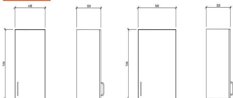
VÄGGSKÅP BVST400V/H ART. NR. 318204-0 (V) ART. NR. 318204-1 (H) ART. NR. 318204-0-12 (V) ART. NR. 318204-1-12 (H)
