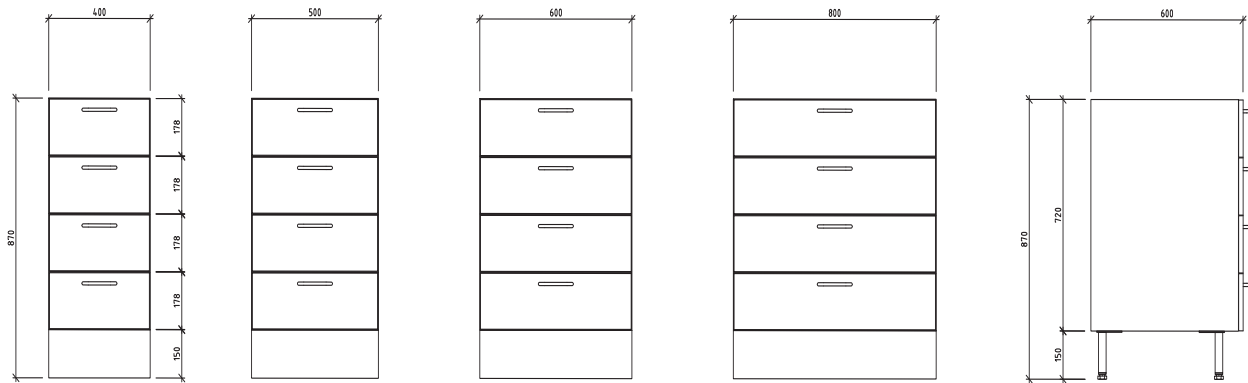
BÄNKSÅP BLH404 ART. NR. 318114-4 ART. NR. 318114-4-12
