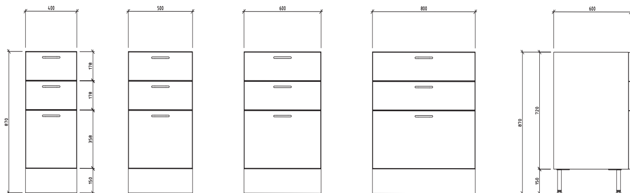
BÄNKSÅP BLH403 ART. NR. 318114-3 ART. NR. 318114-3-12
