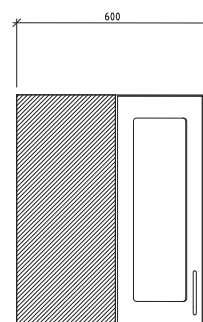
HÖRNVÄGGSKÅP BHVSG600V ART. NR. 3182021-0 (V) ART. NR. 3182021-0-12 (V)
