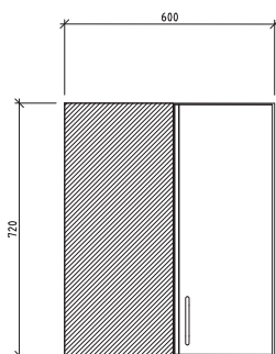
HÖRNVÄGGSKÅP BHVST600H ART. NR. 3182020-1 (H) ART. NR. 3182020-1-12 (H)
