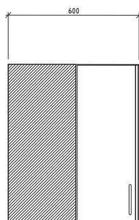
HÖRNVÄGGSKÅP BHVST600V ART. NR. 3182020-0 (V) ART. NR. 3182020-0-12 (V)
