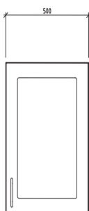
VÄGGSKÅP BVSG500V/H ART. NR. 318215-0 (V) ART. NR. 318215-1 (H) ART. NR. 318215-0-12 (V) ART. NR. 318215-1-12 (H)
