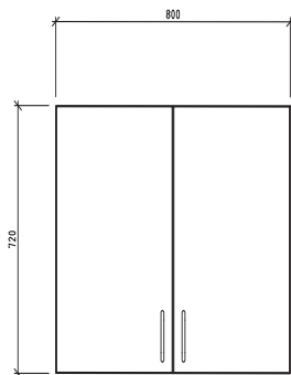
VÄGGSKÅP BVST800 ART. NR. 318208 ART. NR. 318208-12
