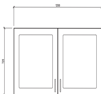
VÄGGSKÅP BVSG1200 ART. NR. 3182112 ART. NR. 3182112-12
