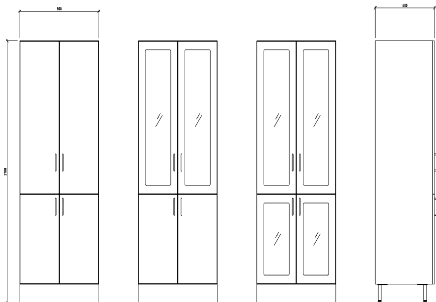
HÖGSKÅP BHSTD800 ART. NR. 318338 ART. NR. 318338-12
